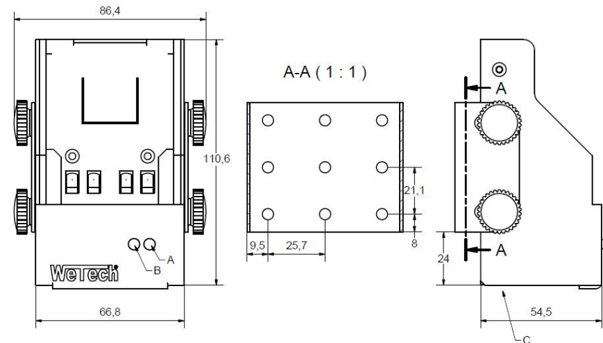
Schemazeichnung WTC636
